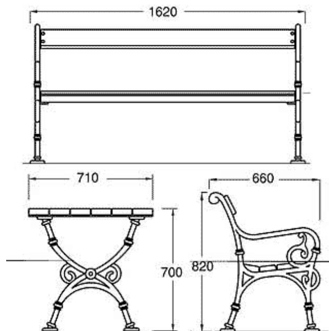
Art. 00 1225/20 1225 - Tavolo con panche modello Vienna - Scheda Tecnica Descrittiva
