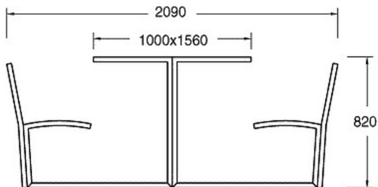
Art. 20 1320 - Tavolo con panche modello Camilla - Scheda Tecnica Descrittiva
